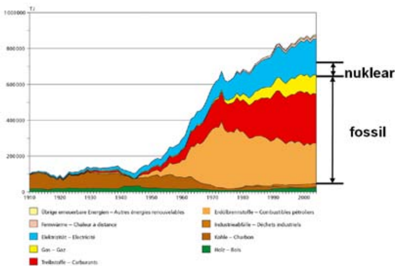
Energieverbrauch der Schweiz, 1910–2004, nach Energieträgern in Terajoule Consommation finale de la Suisse, 1910–2004, selon les agents énergétiques en térajoule
